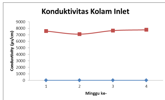
Gambar 2. Monitoring Konduktivitas Air Lindi Inlet
