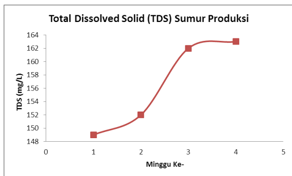
Gambar 10. Monitoring TDS Air Sumur Produksi
