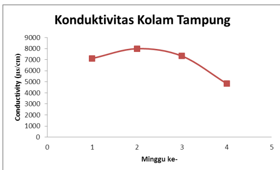
Gambar 5. Monitoring Konduktivitas Air Lindi Kolam Tampung
