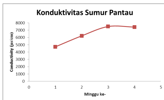
Gambar 8. Monitoring Konduktivitas Air Sumur Pantau
