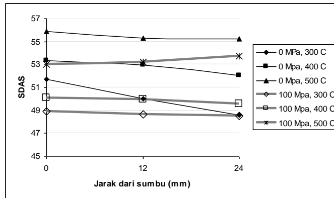
Gambar 9. Ukuran SDAS pada perubahan temperatur cetakan dan jarak pengamatan
