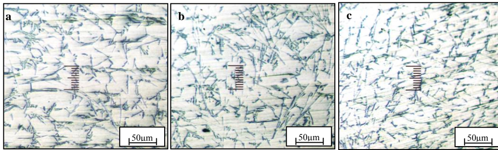
Gambar 6. Struktur mikro spesimen pada temperatur cetakan 300°C, tekanan 100 MPa pada jarak (a). 0 mm, (b). 12 mm, (c). 24 mm dari sumbu
