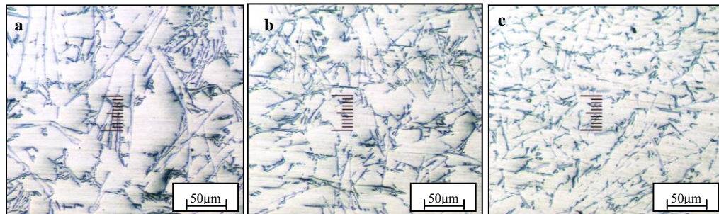
Gambar 7. Struktur mikro spesimen pada temperatur cetakan 400°C, tekanan 100 MPa pada jarak (a). 0 mm, (b). 12 mm, (c). 24 mm dari sumbu
