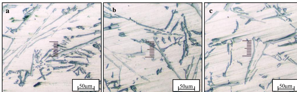
Gambar 5. Struktur mikro spesimen pada temperatur cetakan 500°C, tekanan 0 MPa (pengecoran tuang) pada jarak (a). 0 mm, (b). 12 mm, (c). 24 mm dari sumbu
