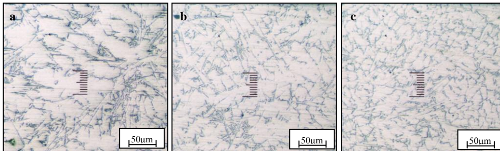
Gambar 4. Struktur mikro spesimen pada temperatur cetakan 300°C, tekanan 0 MPa (pengecoran tuang) pada jarak (a). 0 mm, (b). 12 mm, (c). 24 mm dari sumbu
