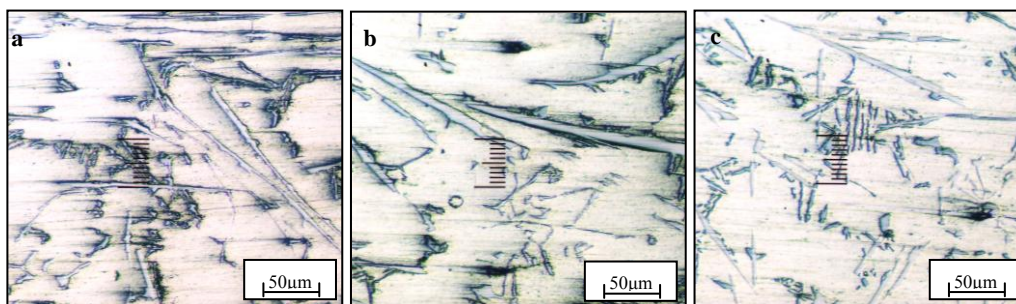
Gambar 8. Struktur mikro spesimen pada temperatur cetakan 500°C tekanan 100 MPa pada jarak (a). 0 mm, (b). 12 mm, (c). 24 mm dari sumbu
