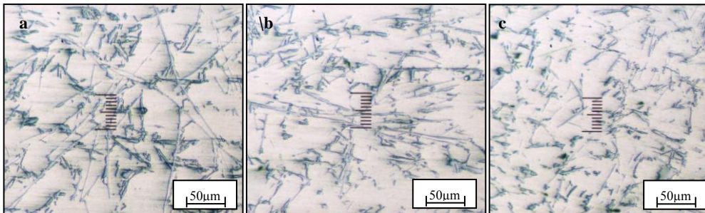
Gambar 3. Struktur mikro spesimen pada temperatur cetakan 400°C, tekanan 0 MPa (pengecoran tuang) pada jarak (a). 0 mm, (b). 12 mm, (c). 24 mm dari sumbu
