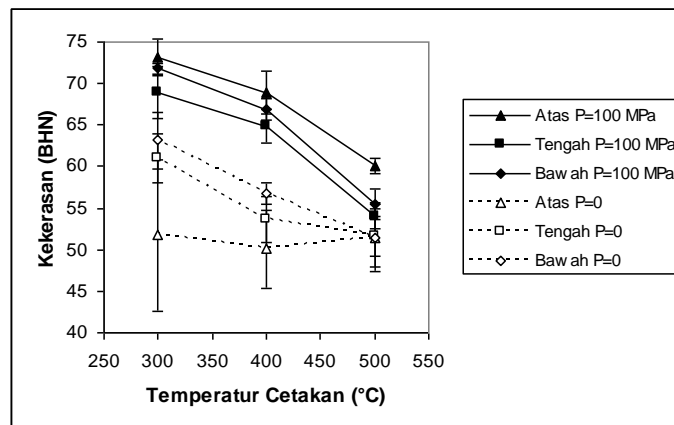
Gambar 10. Harga kekerasan Brinell pada variasi temperatur cetakan
