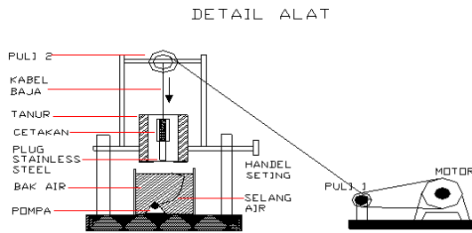
Gambar 1.4 Peralatan pembekuan searah
