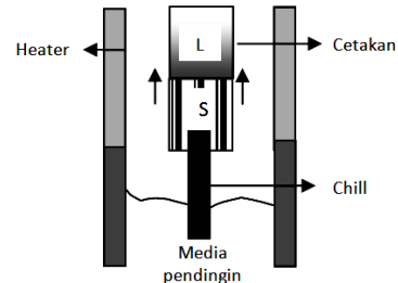
Gambar 1.5 Mekanisme Pembekuan searah
