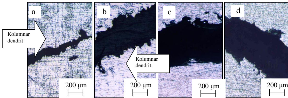
Gambar 1.12 Bentuk patahan tarik pembekuan searah (a) 4,7%Cu, (b) 4,4%Cu, (c) 3,1%Cu, (d) 2,2%Cu.
