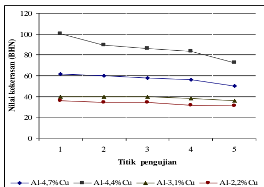
Gambar 1.9 Nilai kekerasan Al-Cu dari pangkal hingga jarak 60 mm
