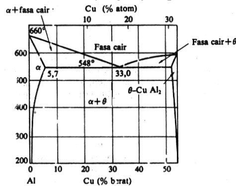
Gambar 1.1 Diagram fase binary Al-Cu (Surdia dan Saito, 1992).
