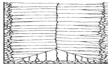
Gambar 1.2 Struktur mikro logam pada cetakan ( Colton, 1992)
