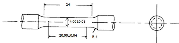
Gambar 1.8 Spesimen uji tarik (ASTM, 2002)
