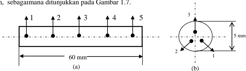
Gambar 1.7 Pengujian kekerasan (a) potongan membujur (b) potongan melintang
