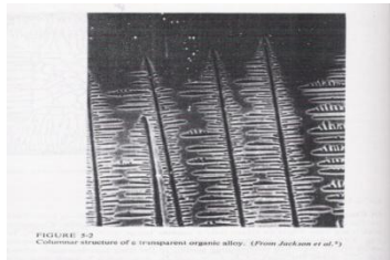
Gambar 1.3 Struktur kolumnar dendrit ( Sindo Kou,1987)
