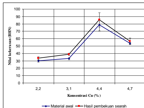
Gambar 1.10 Nilai kekerasan paduan Al-Cu arah membujur
