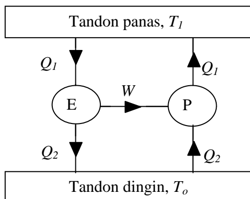
Gambar 2.1 : Mesin kalor ideal, E, pendorong sebuah pendinginan ideal.
