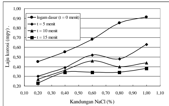
Gambar 4. Pengaruh konsentrasi larutan NaCl dan lama elektroplating terhadap laju korosi baja karbon sedang tanpa lapisan ( raw material ) dan dengan lapisan pada kuat arus 3 \text{ A/dm}^2 , tegangan 12 volt dan suhu 40^\circ \text{C}
