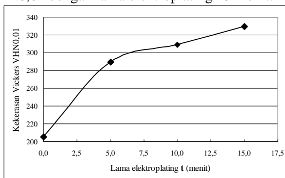
Gambar 3. Pengaruh lama elektroplating terhadap kekerasan Vickers baja karbon sedang pada kuat arus 3 A/dm 2 , tegangan 12 volt dan suhu 40 °C
