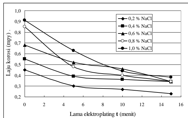
Gambar 5. Pengaruh lama elektroplating dan konsentrasi larutan NaCl terhadap laju korosi baja karbon sedang pada kuat arus 3 \text{ A/dm}^2 , tegangan 12 volt dan temperatur 40^\circ \text{C}
