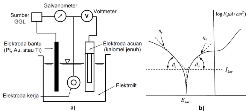
Gambar 2. Skema alat uji korosi tipe sel tiga elektroda (Tretheway dan Chamberlain, 1991)
