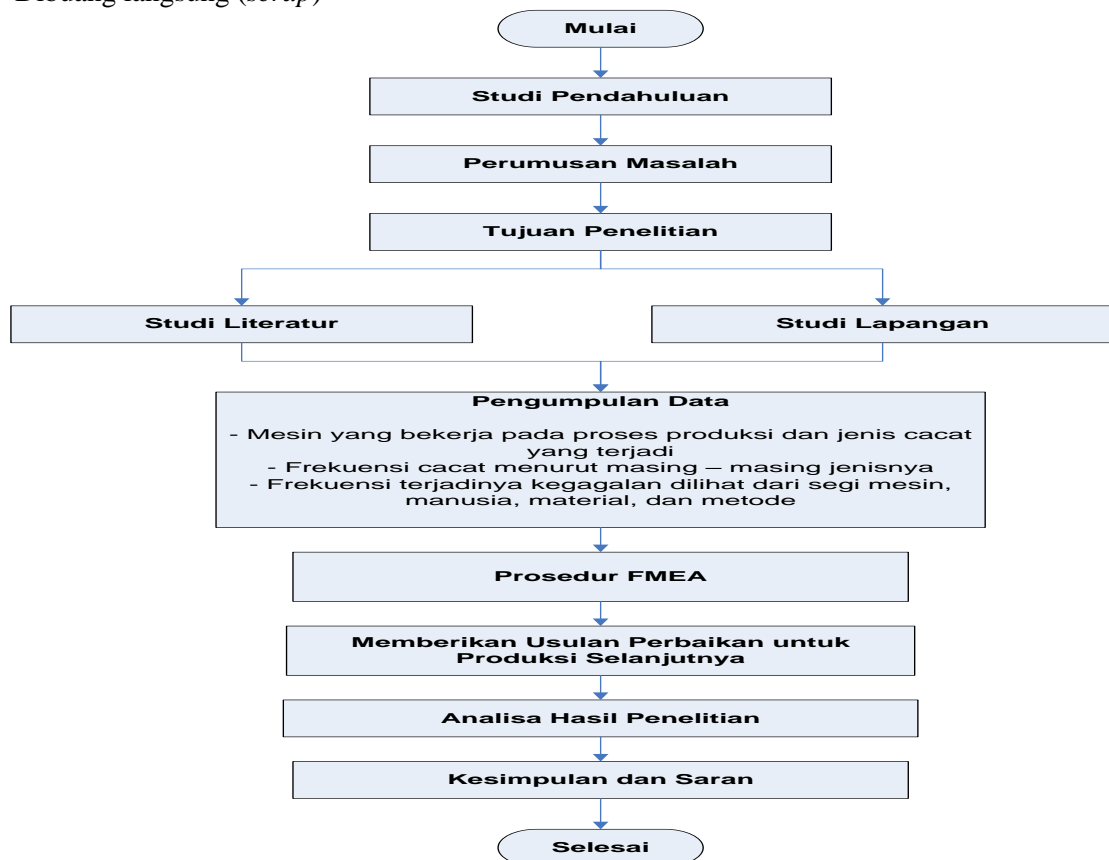
Gambar 1 Metodologi Penelitian
