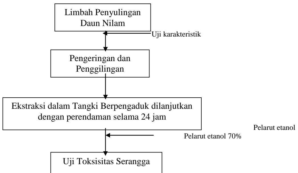
Gambar 2. Diagram Alir Proses Pembuatan Insektisida Nabati
