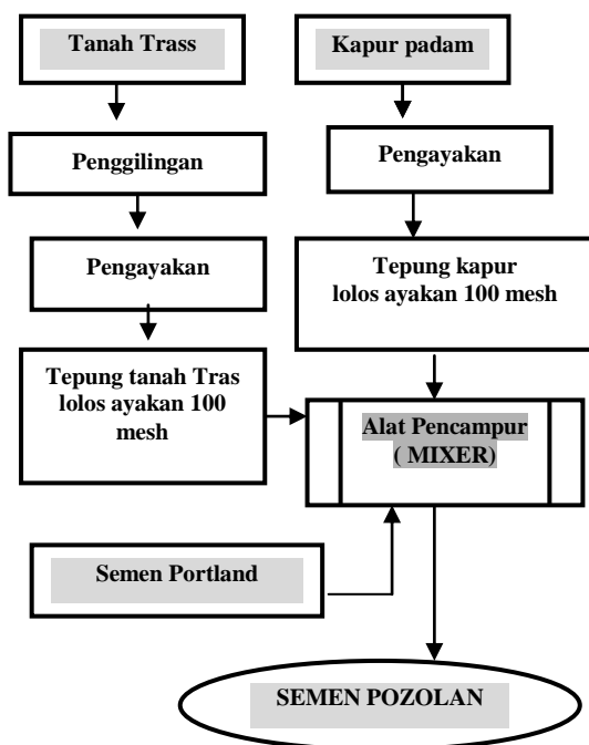
Gambar 1. Proses Pembuatan Semen Pozolan
