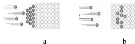
Gambar 3. Modifikasi permukaan; a) pelapisan permukaan, b) difusi elemen ke dalam substrat
